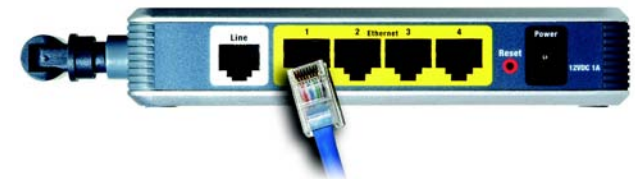
Figure 4-2 : Connexion d'un ordinateur
